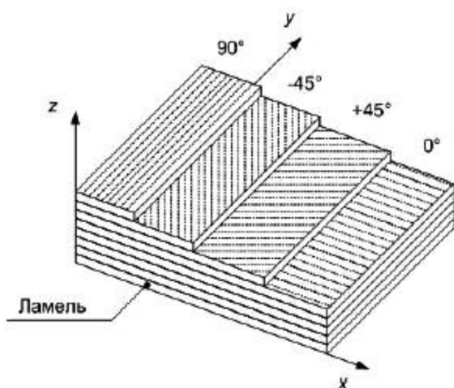
Рисунок 1 - Пример строения ламината конструктивных элементов
